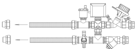
Размеры водяной обвязки для фанкойла
