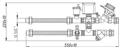
Размеры водяной обвязки для фанкойла
